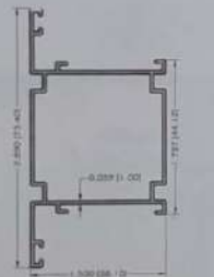
TUBULAR 1 1/2 CON DOBLE ADAPTADOR - ALG 1103
