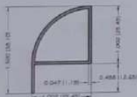
CUARTO DE CIRCULO CON ALETA 1" - T 261
