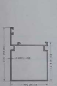
TUBULAR 1 1/2 CON ADAPTADOR - ALG 1101
