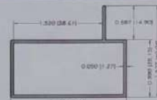
TUBULAR 2X1 CON ALETA SUPERCORRIDA - T 109
