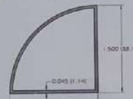
CUARTO DE CIRCULO LISO 1 1/2 - T 232
